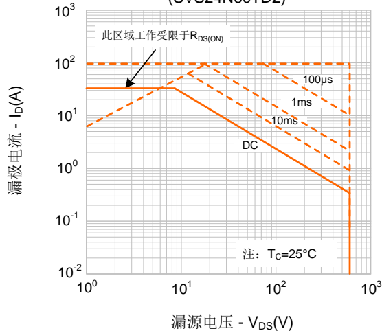
图9-3. 最大安全工作区域 (SVS24N60TD2)
