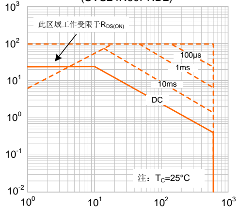
图9-2. 最大安全工作区域 (SVS24N60PND2)
